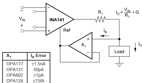
图 6-8. 差分电压至电流转换器
