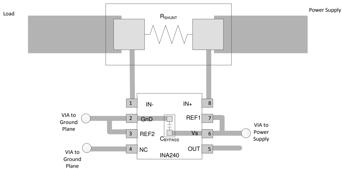
图 11-2. 建议的 SOIC 封装布局
