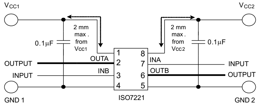
图 8-3. 典型 ISO7221x 电路组装
