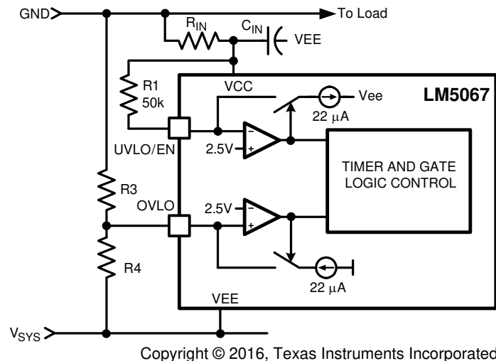
图 9-8. UVLO = POR_{EN}
