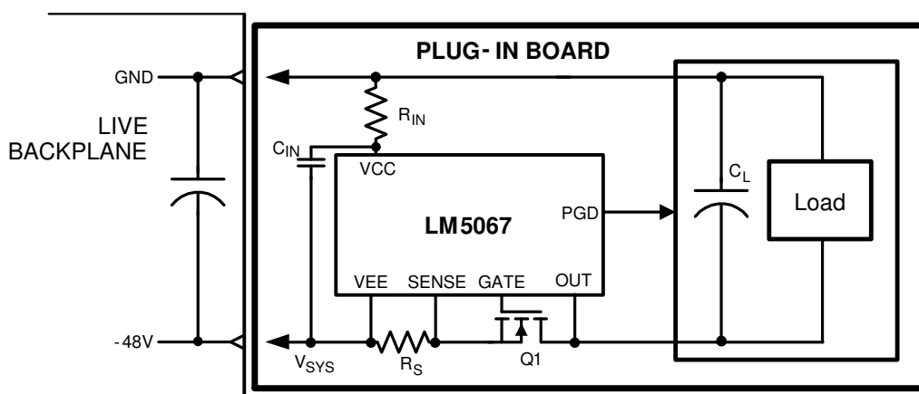
图 8-1. LM5067 Application
