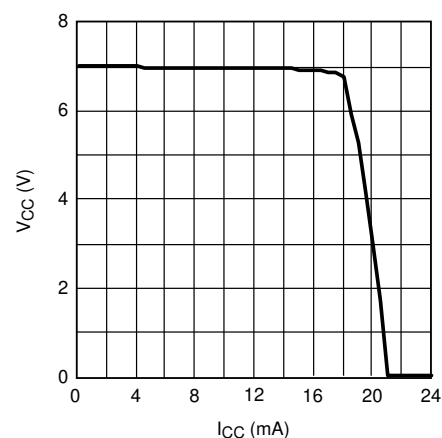
图 5-4. V_{CC} vs I_{CC} V_{IN} = 12\text{V}
