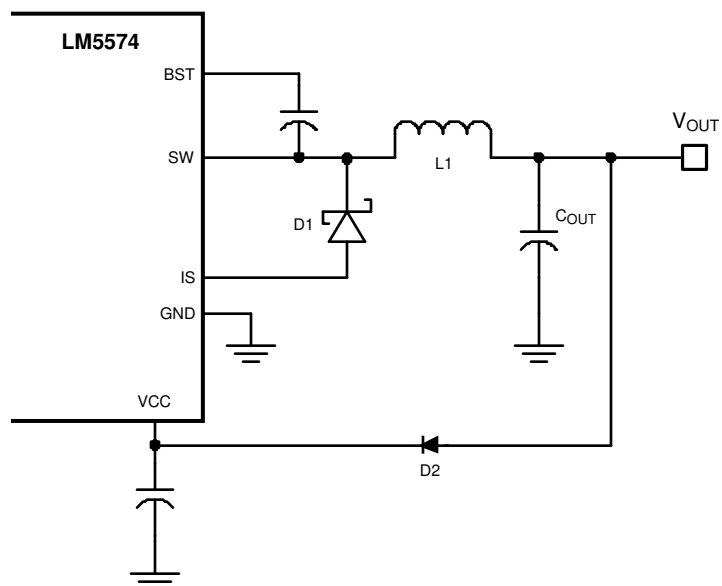
图 7-6. Vcc Bias From Vout for 8V &lt; Vout &lt; 14V
