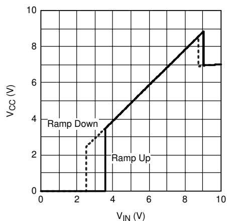
图 5-5. V_{CC} vs V_{IN} R_L = 7\text{k}\Omega
