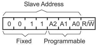
图 7-7. PCA9557 Address
