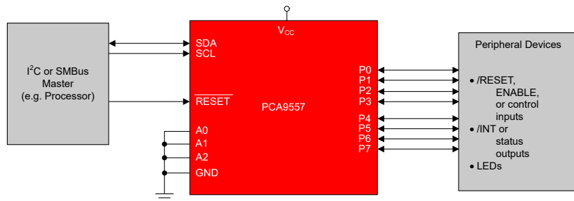
逻辑图
