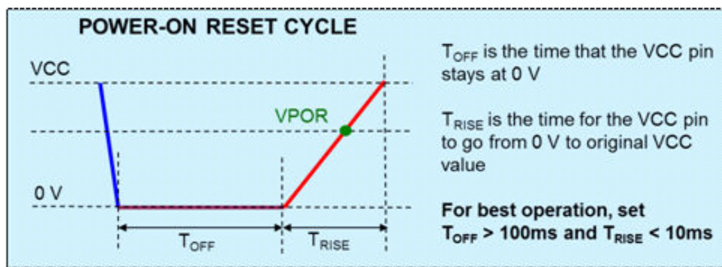
图 8-4. Power-On Reset
