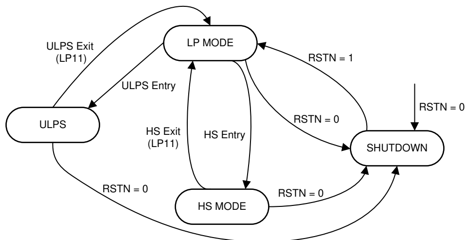
图 6-2. Functional Modes
