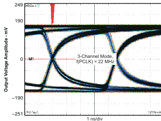
图 6-15. VGA 3-channel Output Waveform
