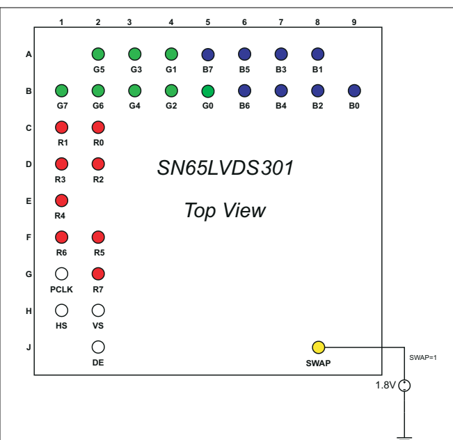
图 8-3. SWAP PIN = 1
