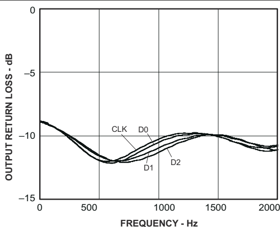
图 6-19. Output Return Loss
