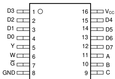
D 或 PW 封装 16 引脚 SOIC 或 TSSOP 顶视图
