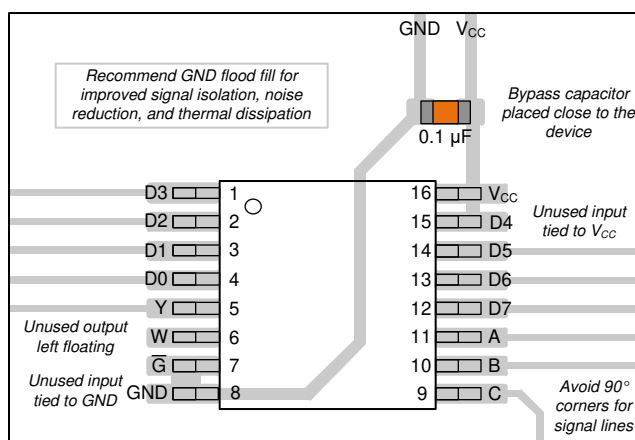
图 8-3. SN74HCS151 的示例布局。
