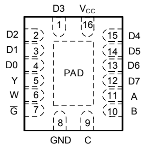
WBQB 封装 16 引脚 WQFN 俯视图
