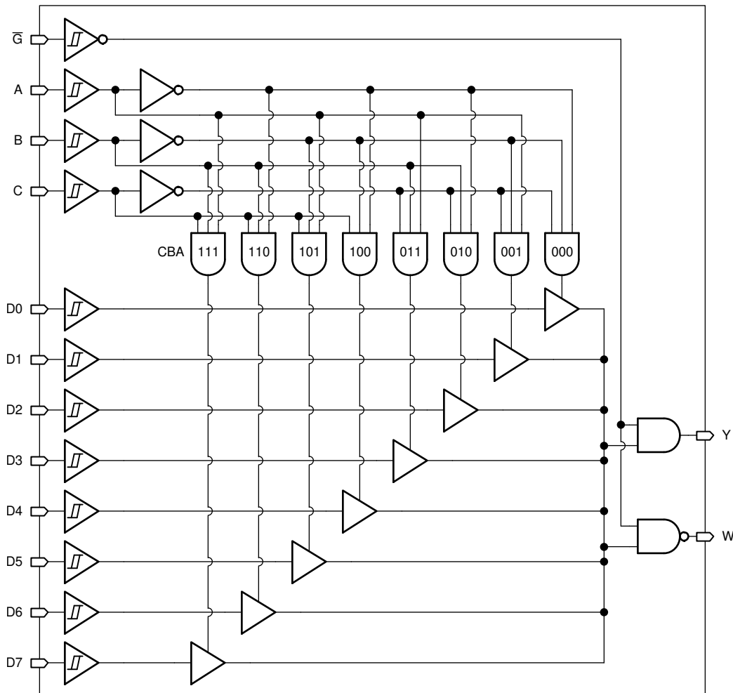
图 7-1. SN74HCS151 的逻辑图 (正逻辑)
