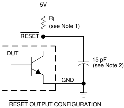
图 7-1. RESET Output Configuration
