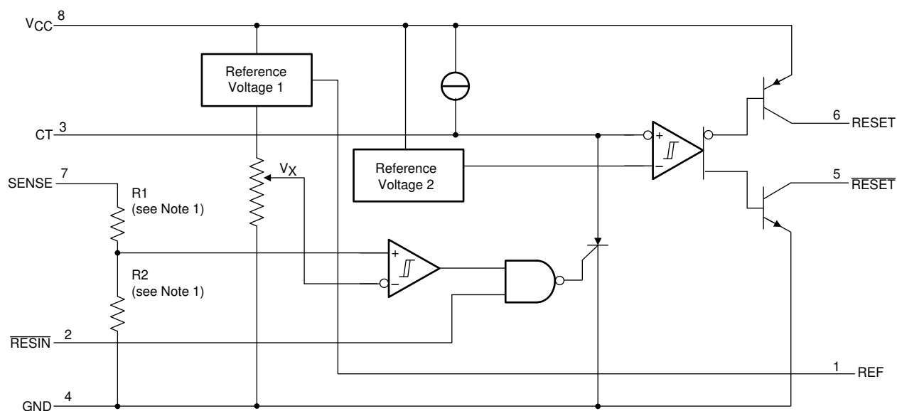
功能方框图
