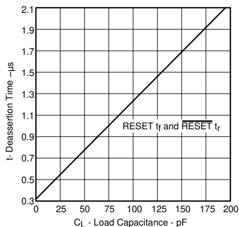
图 6-6. Deassertion Time vs Load Capacitance
