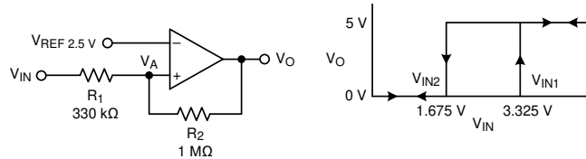
图 7-5. 具有迟滞功能的同相配置
