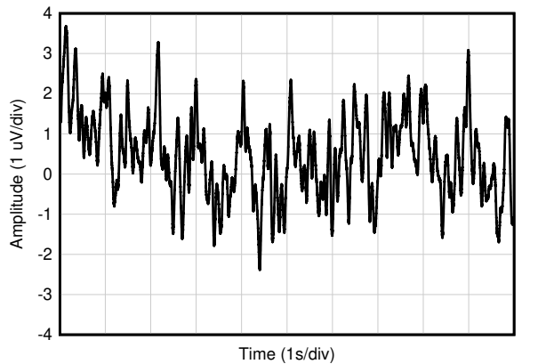
图 7-21. 0.1Hz 至 10Hz 时域电压噪声
