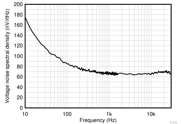
图 7-22. 输入电压噪声频谱密度
