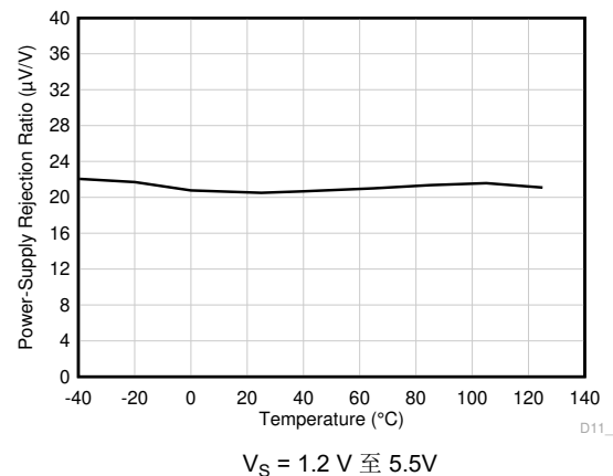
图 7-18. 直流 PSRR 与温度间的关系
