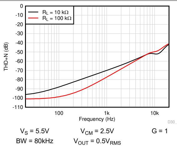
图 7-23. THD+N 与频率间的关系
