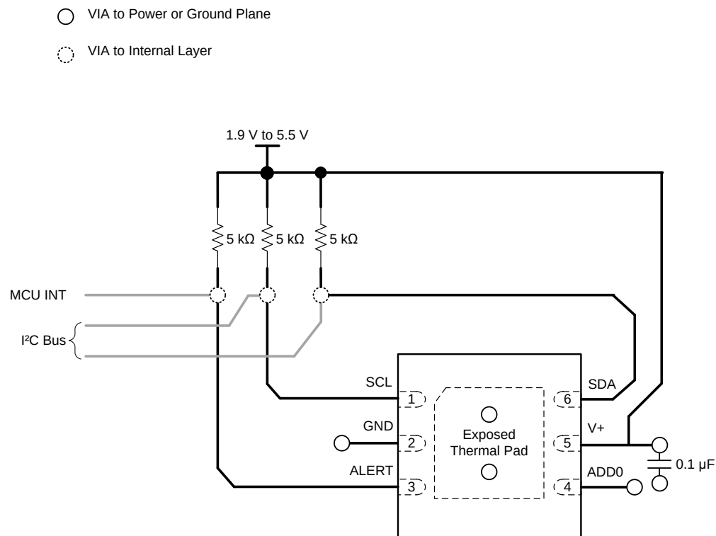
图 45. Layout Recommendation
