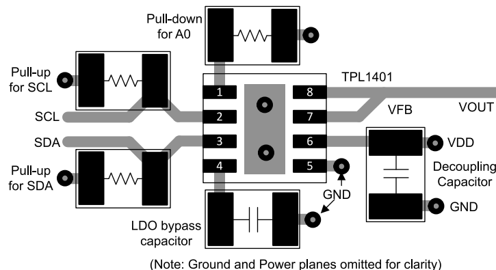
图 10-1. Layout Example
