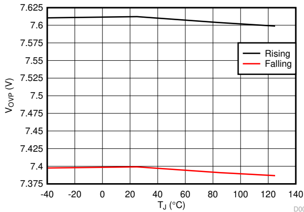
TPS259803x 型号
