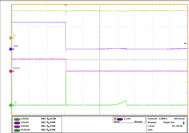
图 6-29. 断路器 - 自动重试
