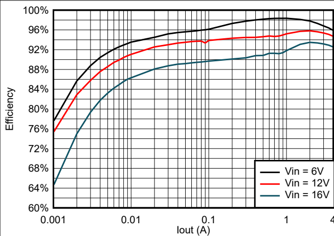
图 6-17. TPS564242 在 5V OUT 且使用 1.8 µH 电感器时的效率
