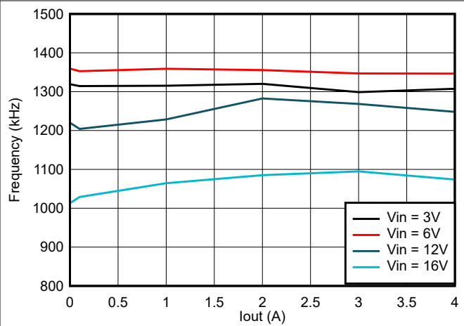
图 8-3. TPS564247 频率与负载间的关系
