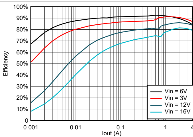
图 6-13. TPS564242 在 1.05V OUT 且使用 0.82 µH 电感器时的效率
