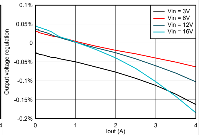
图 8-5. TPS564247 负载调整率与负载间的关系
