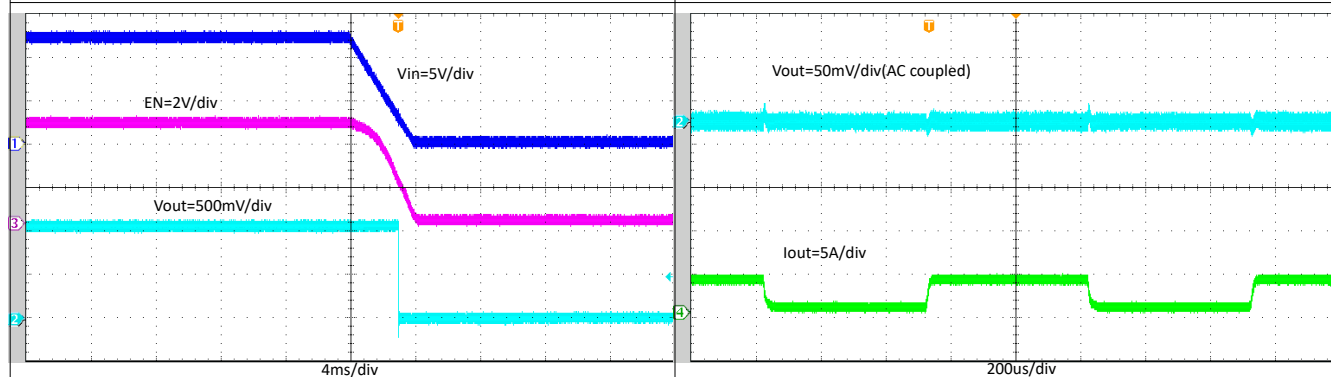
图 8-14. 在 V_{IN} 下降时启动, I_{OUT} = 4A
