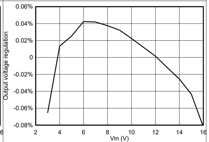
图 8-7. TPS564247 线性调整率与 V_{IN} 间的关系 (4A 负载)
