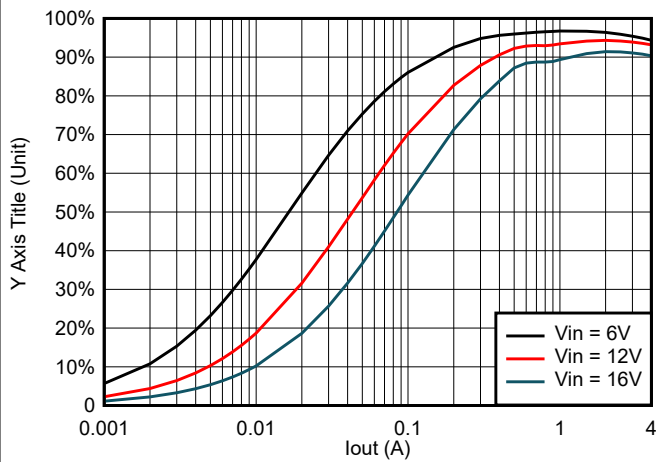
图 6-16. TPS564247 在 3.3V OUT 且使用 1.5 µH 电感器时的效率
