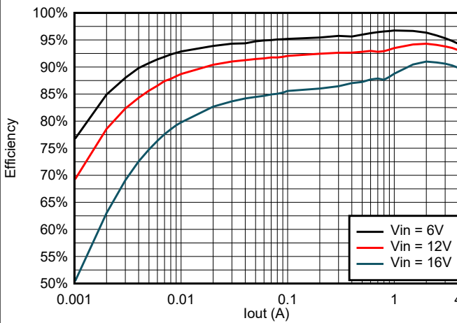
图 6-15. TPS564242 在 3.3V OUT 且使用 1.5 µH 电感器时的效率
