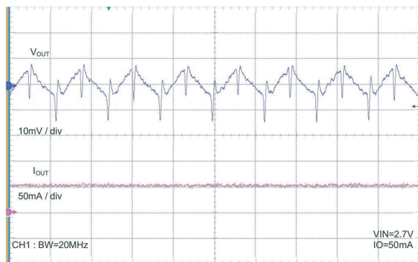
图 7-10. 输出纹波电压 (正常模式) V_{IN} = 2.7V , I_O = 50mA
