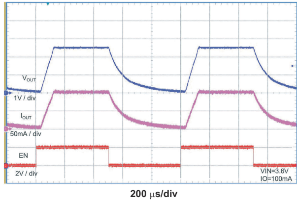
图 7-15. 使能/禁用 V_{IN} = 3.6V , I_O = 100mA
