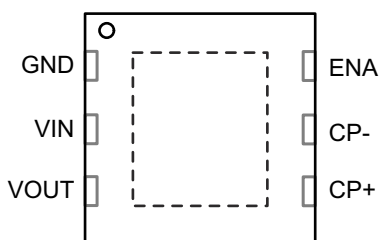
图 4-1. DRV 封装 6 引脚 WSON (俯视图)
