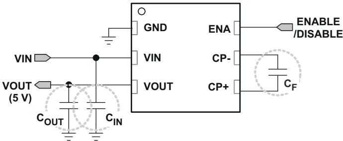
图 7-2. 电容器
