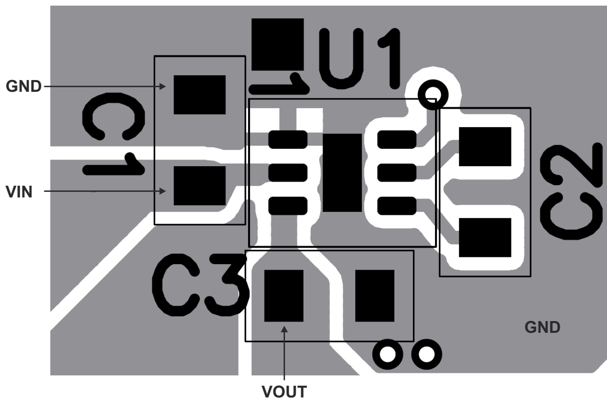
图 7-18. 建议的 PCB 布局
