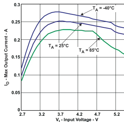
图 5-2. 不同温度下最大输出电流与输入电压的关系
