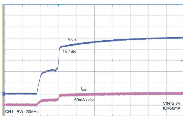
图 7-12. 上电 V_{IN} = 2.7V , I_O = 50mA
