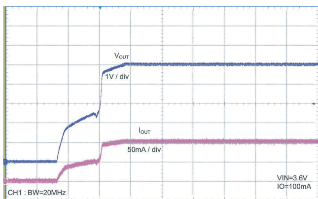
图 7-13. 上电 V_{IN} = 3.6V , I_O = 100mA
