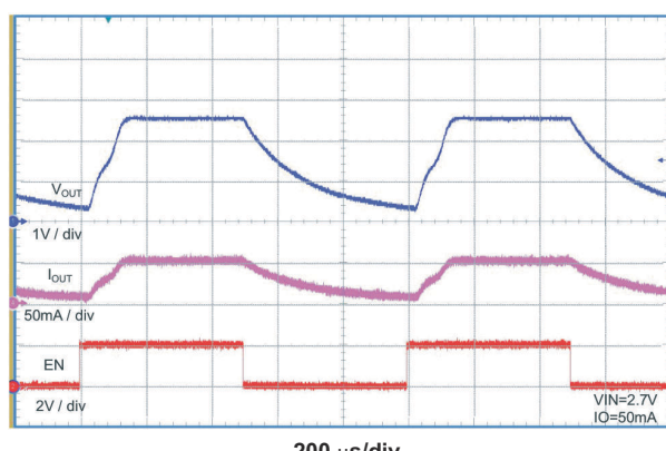
图 7-14. 使能/禁用 V_{IN} = 2.7V , I_O = 50mA
