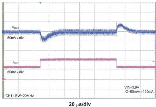
图 7-7. V_{IN} = 3.6V 、 I_O 从 60mA 变为 100mA 时的负载瞬态响应
