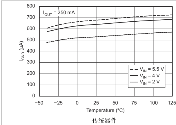
图 5-13. 接地引脚电流与温度间的关系
