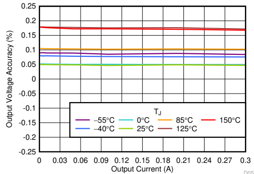
图 6-2. Output Accuracy vs I_{OUT}
