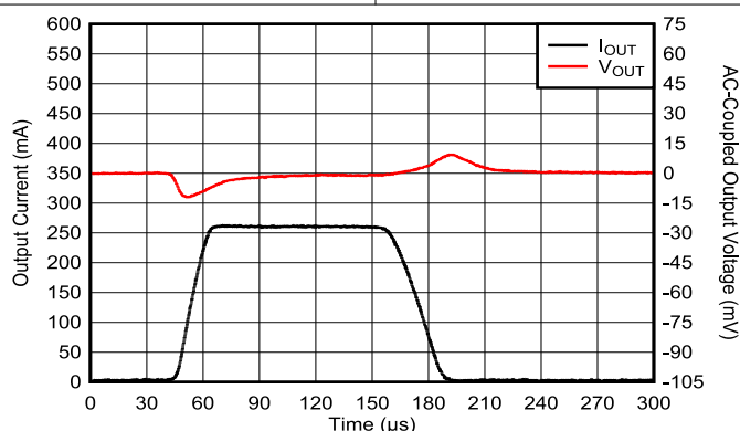
图 8-7. TPS794 负载瞬态响应
