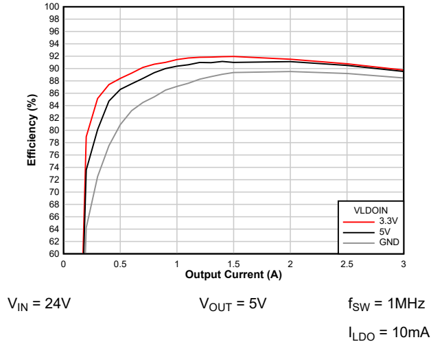
图 8-8. 通过 VLDIOIN 实现的效率提升 ( V_{OUT} = 5V )
