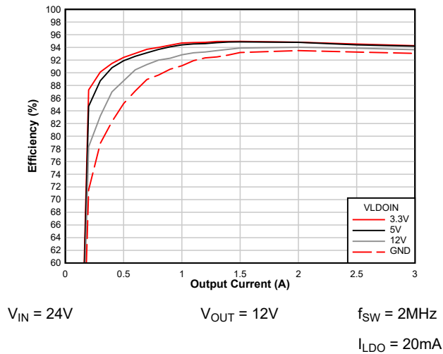
图 8-9. 通过 VLDIOIN 实现的效率提升 ( V_{OUT} = 12V )
