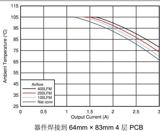
图 7-23. 安全工作区 V_{OUT} = 5.0V , f_{sw} = 1MHz
