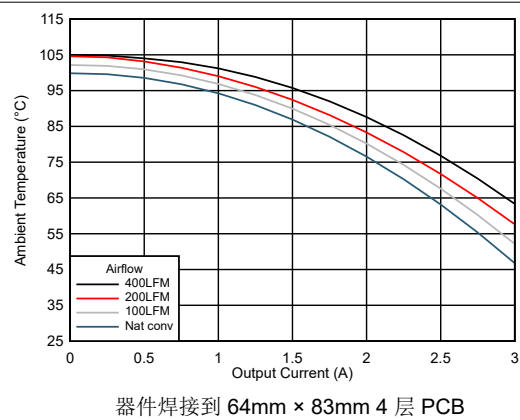
图 7-24. 安全工作区 V_{OUT} = 12V , f_{sw} = 2MHz
