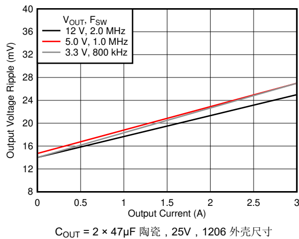
图 7-21. 输出电压纹波
