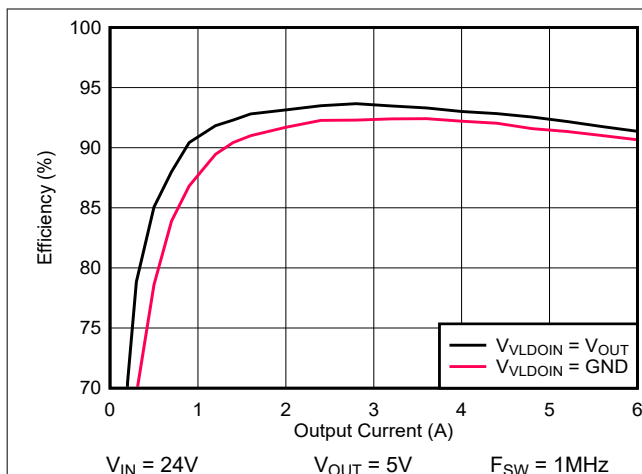
图 8-5. 通过外部偏置提高效率
