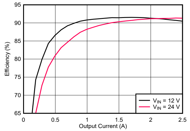
图 9-14. 效率
