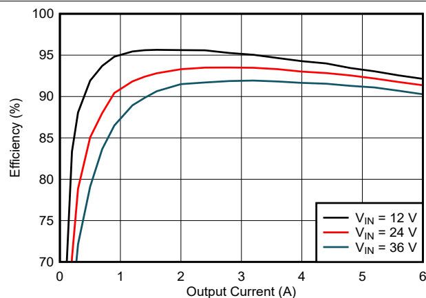
图 9-2. 效率
