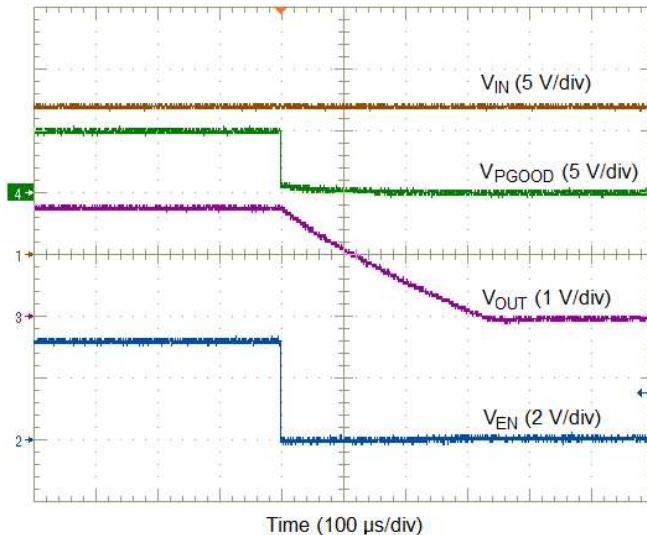
图 13. Enable Turnoff
