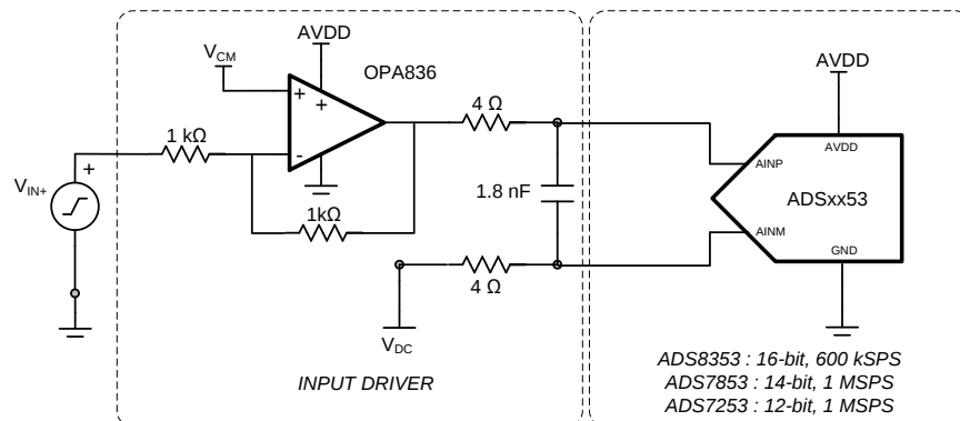
典型应用图
