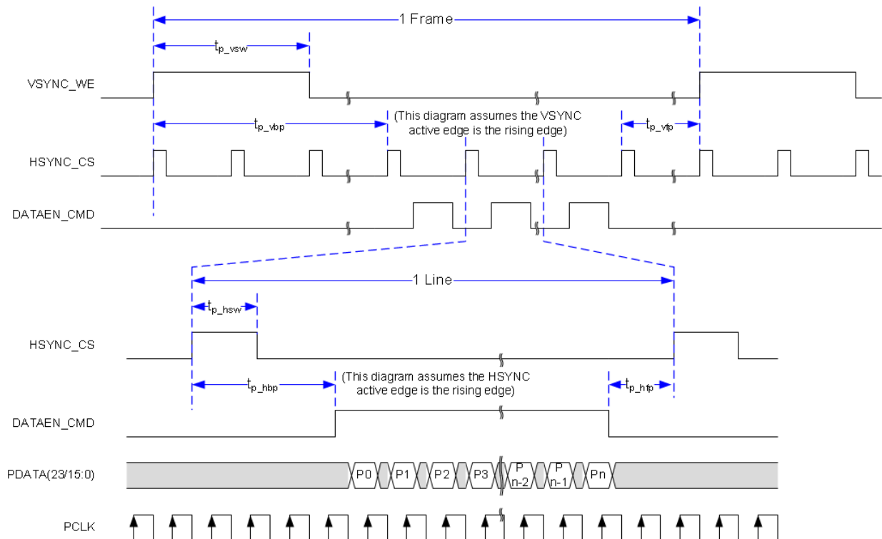
图 5-10. 源帧时序
