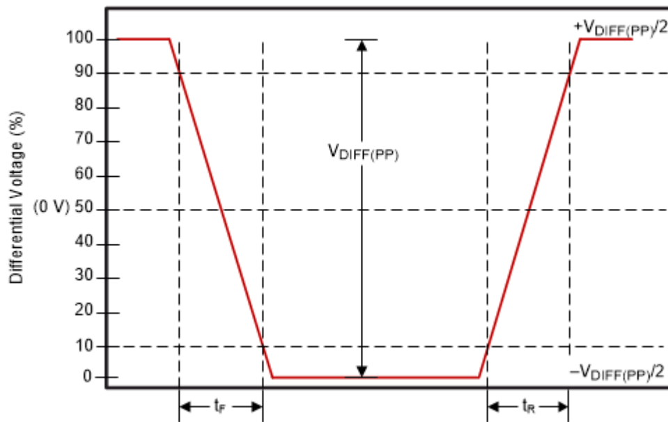
图 5-15. DMD 低速差分时序参数
