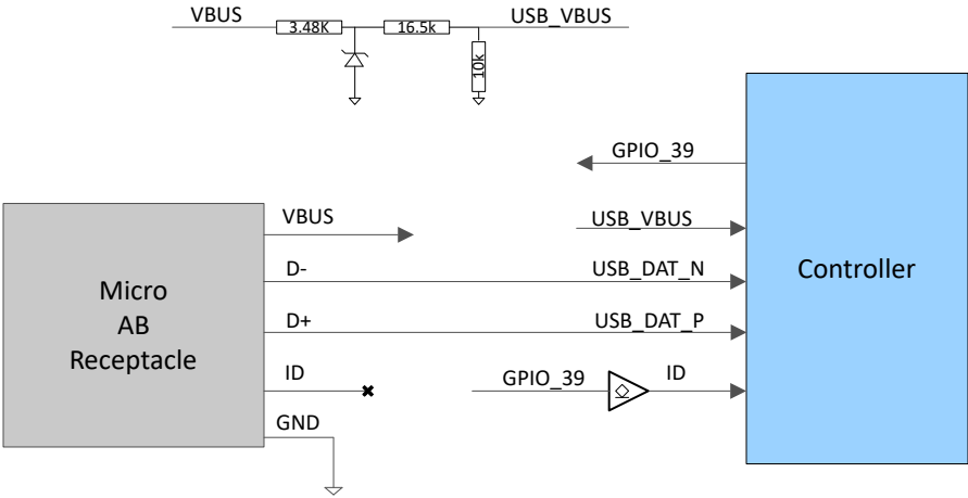
图 5-5. DLPC8445 控制器的 USB 示例
