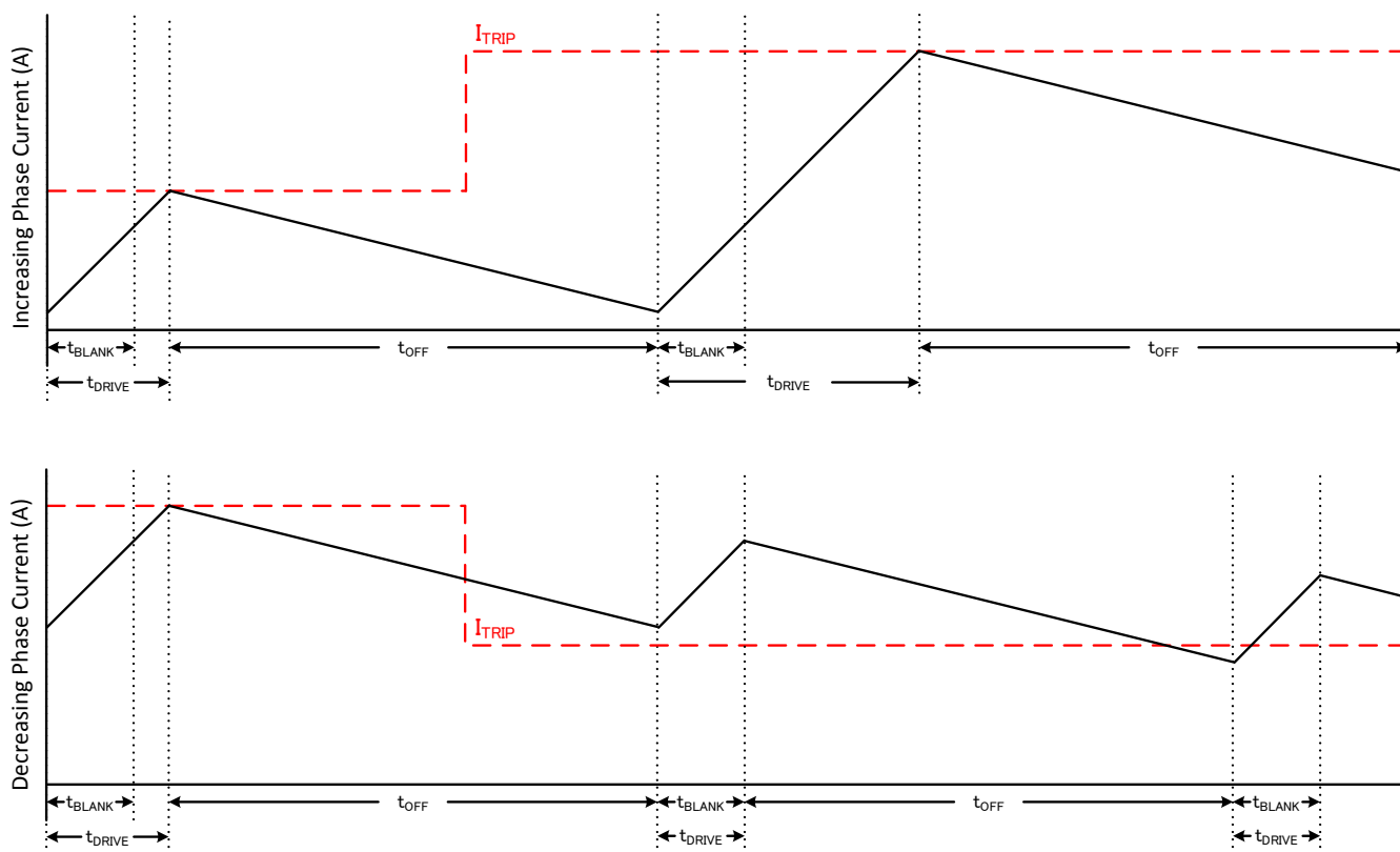
图 7-13. 慢速衰减模式
