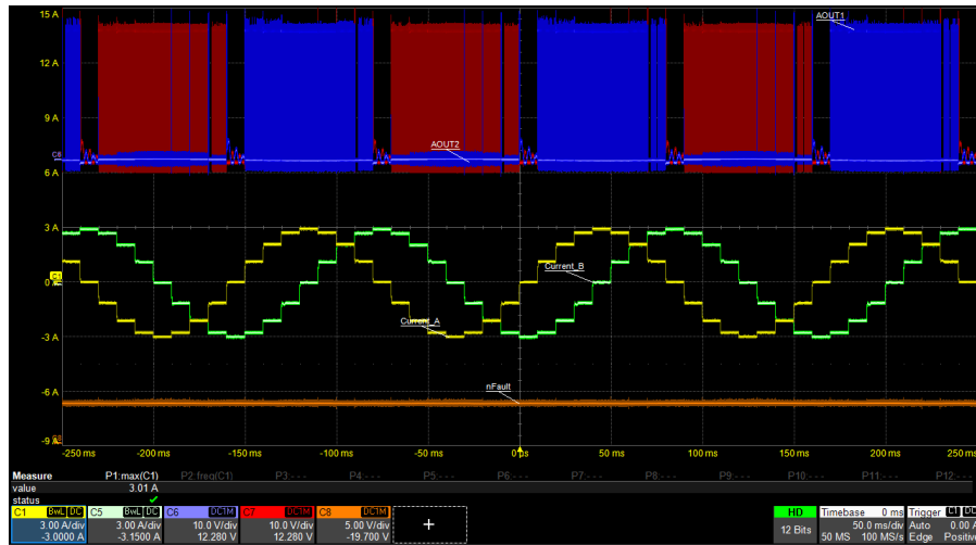
图 8-4. 在 100pps、 I_{FS} = 3\text{ A} 时为 1/4 微步进
