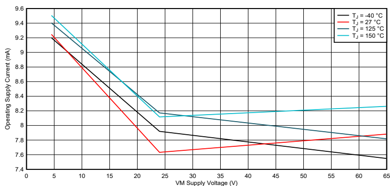
图 6-5. 工作电源电流，VCC = DVDD
