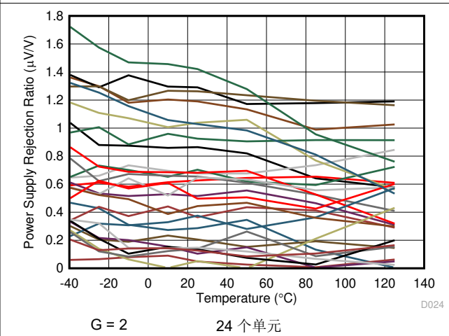
图 7-24. PSRR 与温度间的关系
