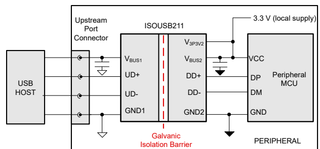
应用示意图
