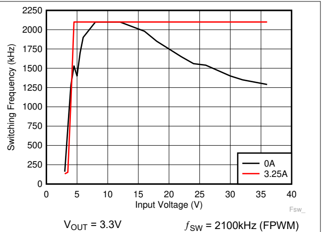
图 8-15. 开关频率与输入电压间的关系
