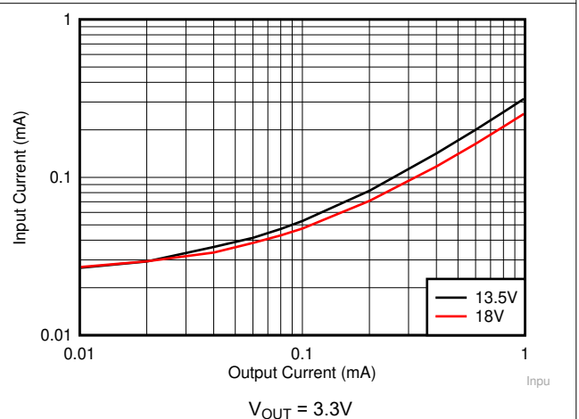
图 8-19. 输入电源电流与输出电流间的关系
