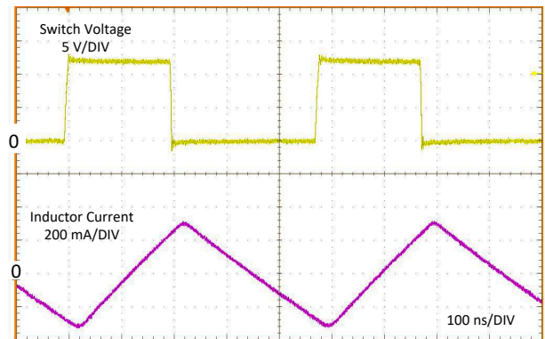
图 7-7. 没有展频的典型 PWM 开关波形, V_{IN} = 12V , V_{OUT} = 5V , I_{OUT} = 3.25A , f_{SW} = 2100kHz
