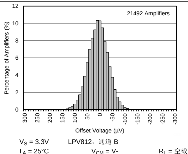
图 8. LPV812 的失调电压分布, 通道 B
