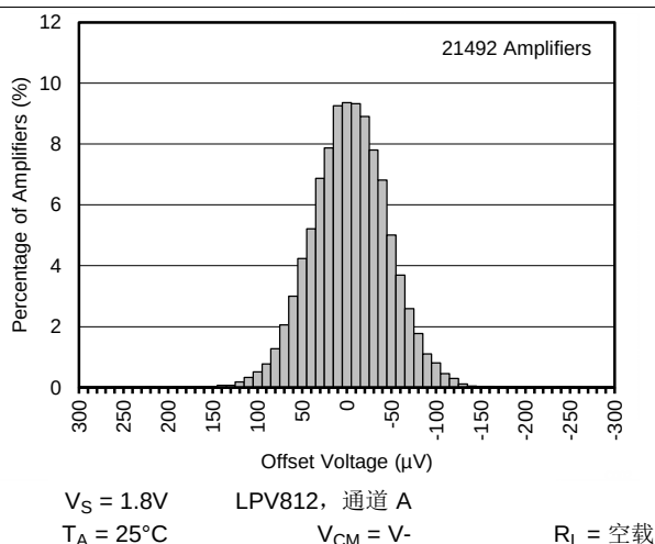
图 5. LPV812 的失调电压分布, 通道 A
