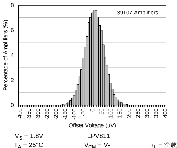
图 3. LPV811 的失调电压分布
