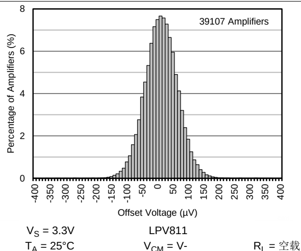
图 4. LPV811 的失调电压分布
