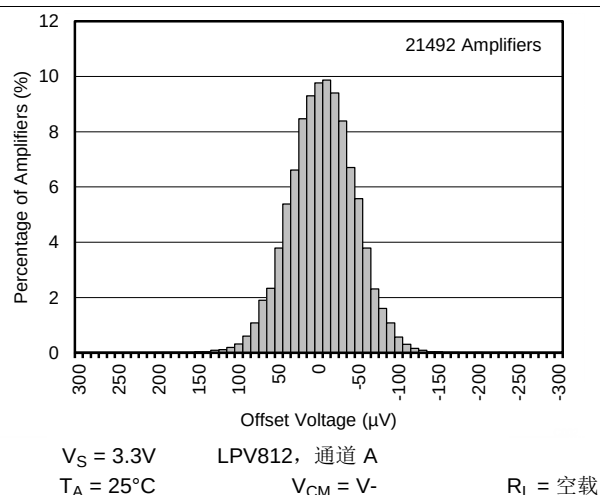
图 6. LPV812 的失调电压分布, 通道 A
