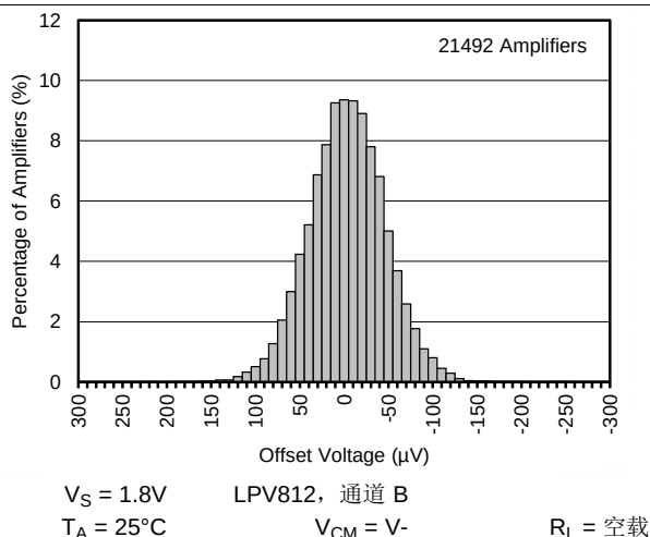
图 7. LPV812 的失调电压分布, 通道 B
