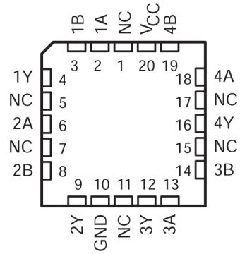
图 3-2. SN54AC86 FK Package (Top View)
