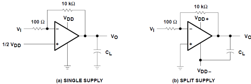
图 5-3. 100 倍增益反相放大器
