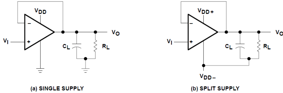
图 5-1. 单位增益放大器
