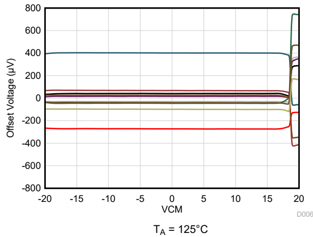
图 4-7. 失调电压与共模电压间的关系
