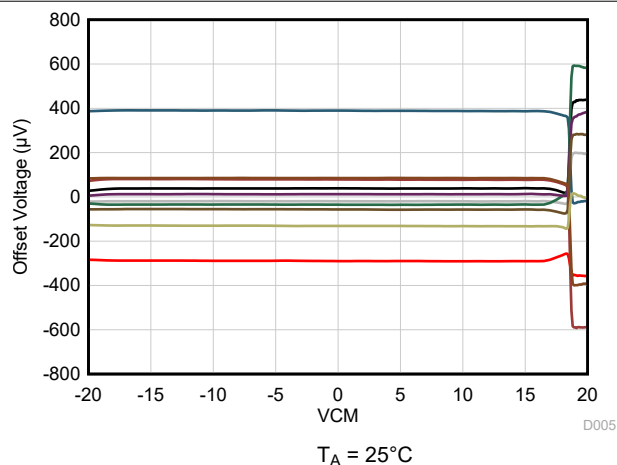
图 4-5. 失调电压与共模电压间的关系
