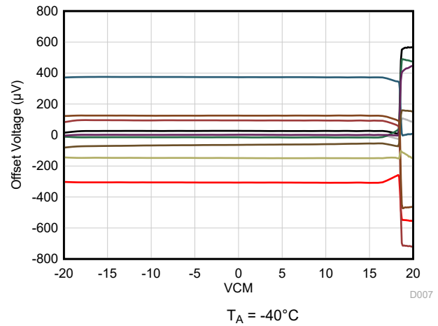
图 4-8. 失调电压与共模电压间的关系
