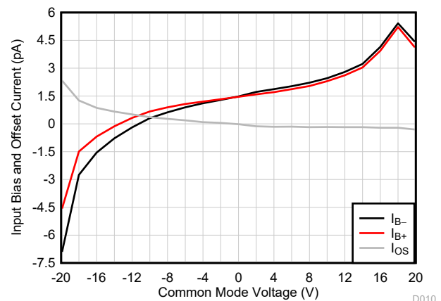
图 4-12. 输入偏置电流与共模电压间的关系
