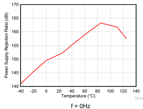
图 4-18. PSRR 与温度间的关系 (dB)
