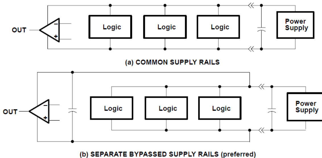
图 6-3. 公共电源导轨与独立电源导轨
