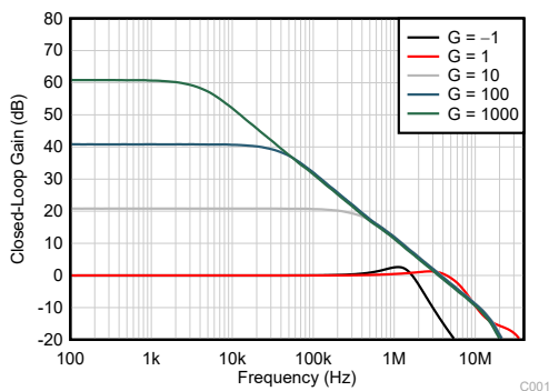
图 4-11. 闭环增益与频率间的关系
