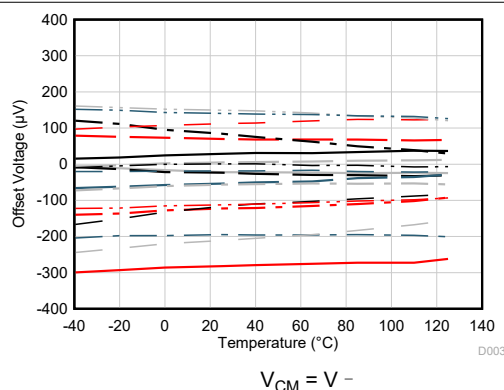
图 4-4. 失调电压与温度间的关系
