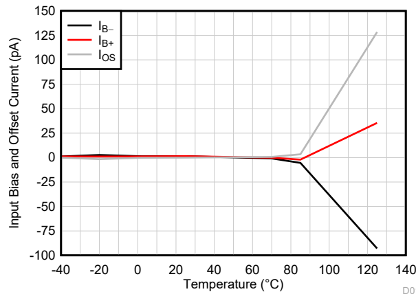
图 4-13. 输入偏置电流与温度间的关系
