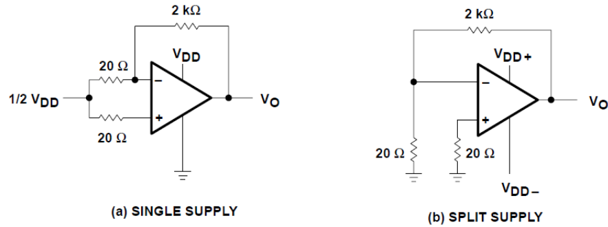
图 5-2. 噪声测试电路
