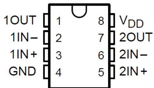
图 3-1. D、JG、P 或 PW 封装 (顶视图)
