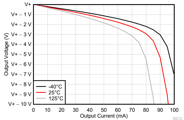
图 4-14. 输出电压摆幅与输出电流 (拉电流) 间的关系
