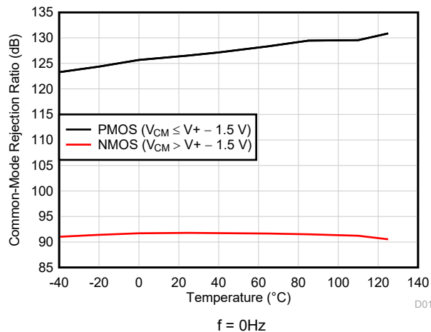
图 4-17. CMRR 与温度间的关系 (dB)
