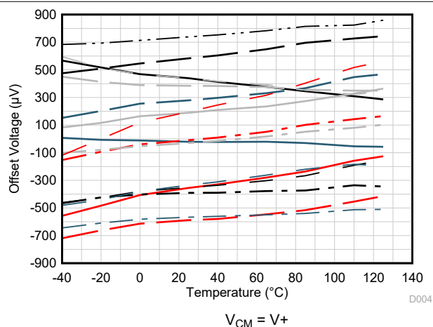
图 4-3. 失调电压与温度间的关系
