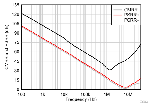
图 4-16. CMRR 和 PSRR 与频率间的关系
