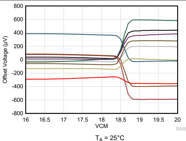
图 4-6. 失调电压与共模电压间的关系 (切换区域)
