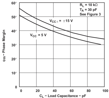
图 6-49. TLE2021 相位裕度与负载电容间的关系
