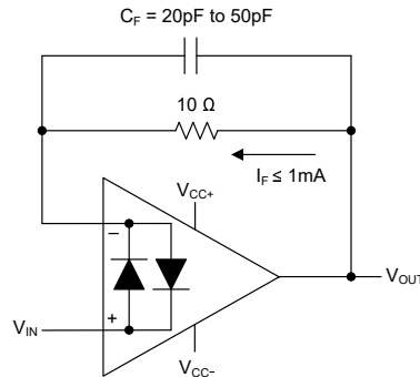
图 7-1. 电压输出器
