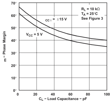
图 6-50. TLE2022 和 TLE2024 相位裕度与负载电容间的关系
