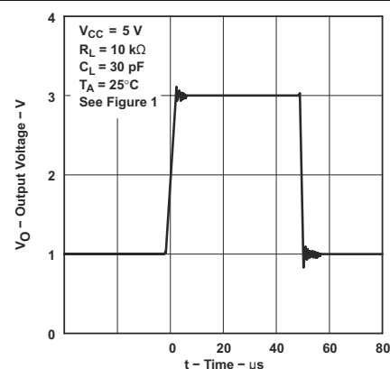
图 6-34. 电压输出器小信号脉冲响应
