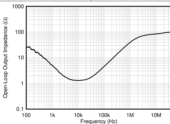
图 6-17. 开环输出阻抗与频率间的关系
