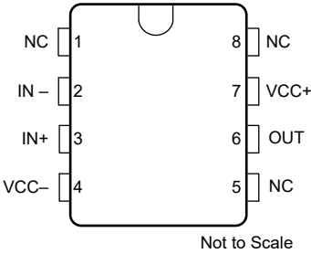
图 5-1. TLE2081D 或 P 封装 ( 顶视图 )
