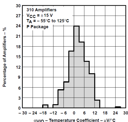
图 6-5. TLE2082 输入失调电压温度系数的分布
