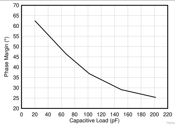
图 6-12. 相位裕度与负载电容间的关系
