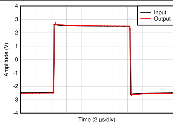
图 6-13. 同相大信号脉冲响应
