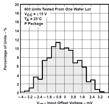
图 6-2. TLE2082 输入失调电压的分布
