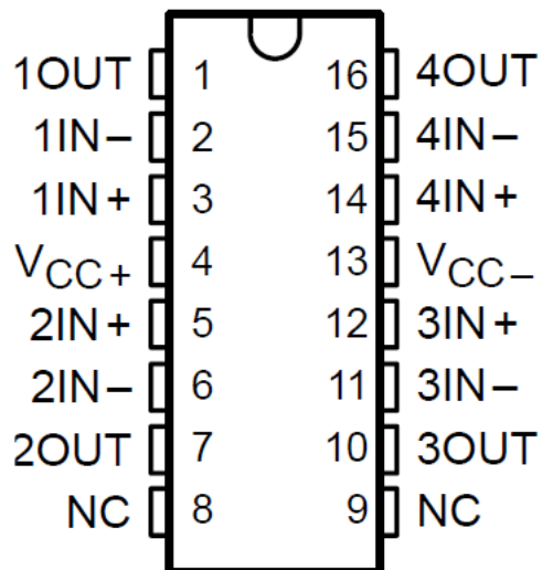
图 5-4. TLE2084 DW 封装
