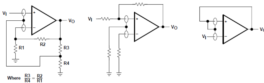
图 7-1. 使用防护环
