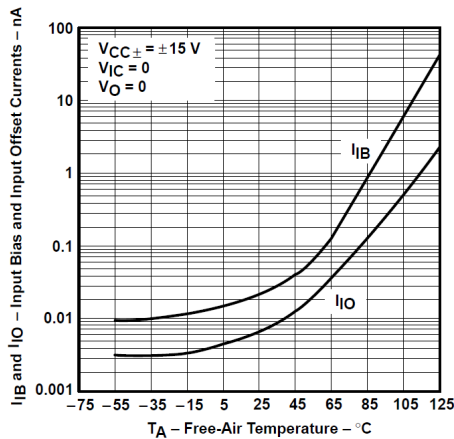
图 6-9. TLE2081 和 TLE2082 输入偏置电流和输入偏移电流与自然通风温度间的关系
