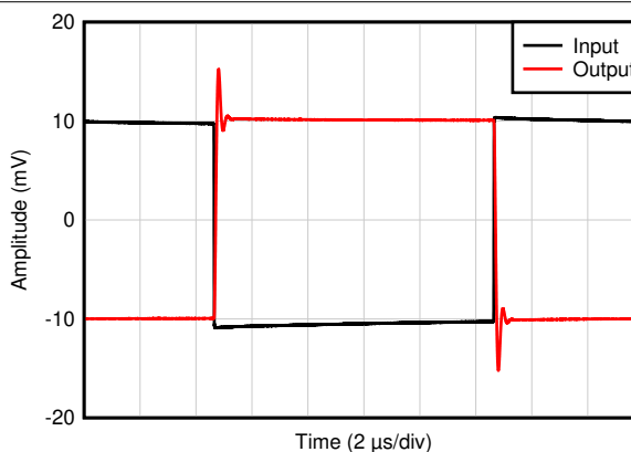
图 6-16. 小信号脉冲响应
