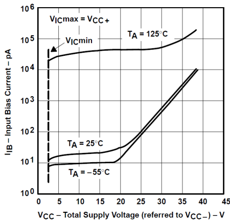
图 6-11. 输入偏置电流与总电源电压间的关系
