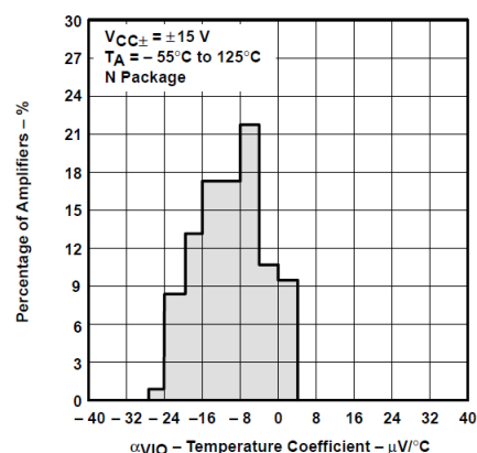
图 6-6. TLE2084 输入失调电压温度系数的分布
