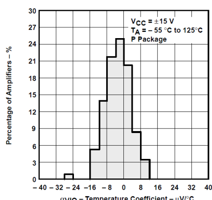
图 6-4. TLE2081 输入失调电压温度系数的分布
