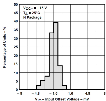
图 6-3. TLE2084 输入失调电压的分布
