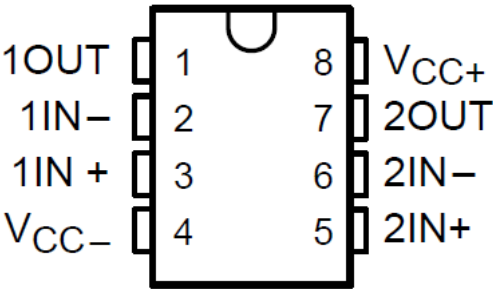
图 5-2. TLE2082D 或 P 封装 ( 顶视图 )
