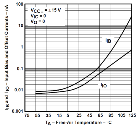
图 6-10. TLE2084 输入偏置电流和输入偏移电流与自然通风温度间的关系
