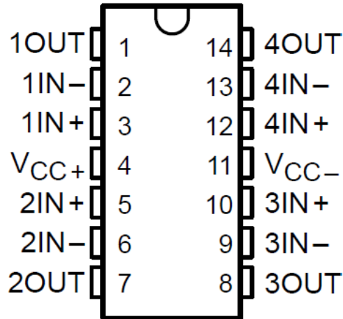
图 5-3. TLE2084N 封装 (顶视图)
