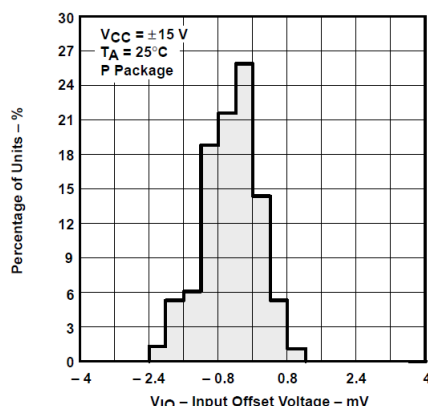
图 6-1. TLE2081 输入失调电压的分布
