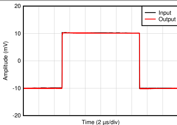
图 6-15. 小信号脉冲响应
