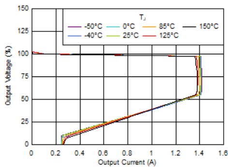
图 5-4. 负载调节 (可调节输出, 新芯片)
