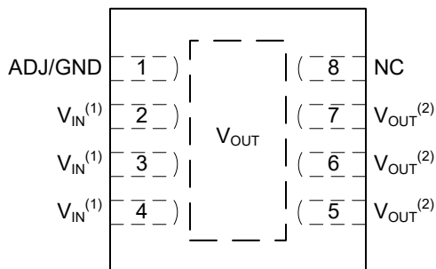
图 4-5. DRJ 封装，8 引脚 WSON (俯视图)
