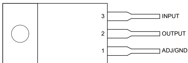
图 4-2. KCT 和 KCS 封装，3 引脚 TO-220 (俯视图)
