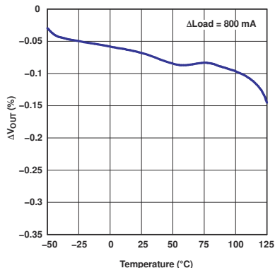
图 5-1. 负载调整 (旧芯片)
