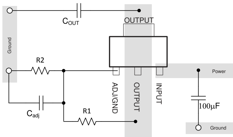
图 7-11. 布局示例
