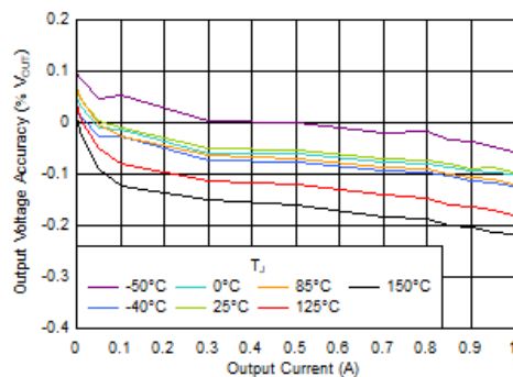
图 5-2. V_{OUT} 精度与 I_{OUT} 之间的关系 (固定输出, 新芯片)
