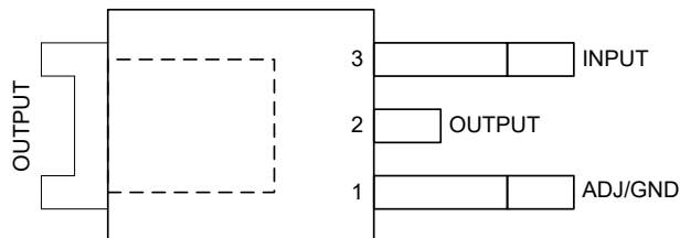
图 4-4. KVU 封装，3 引脚 TO-252 (顶视图)
