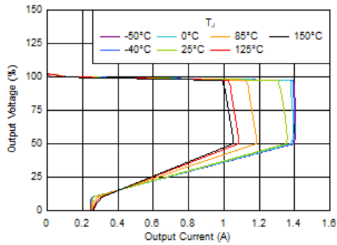
图 5-7. 折返电流限制与温度之间的关系 (固定输出, 新芯片)
