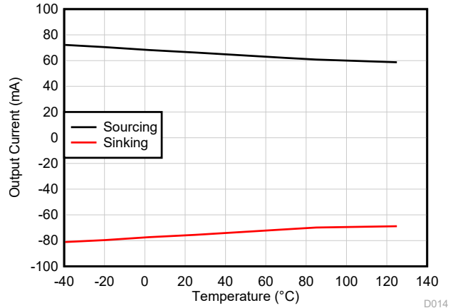
图 6-38. 短路电流与温度之间的关系
