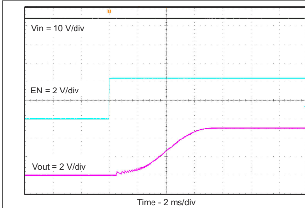
图 7-14. 相对于 EN 的启动
