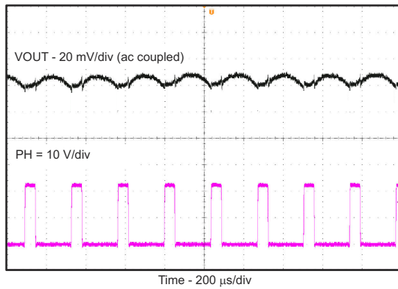
图 7-8. 输出电压纹波
