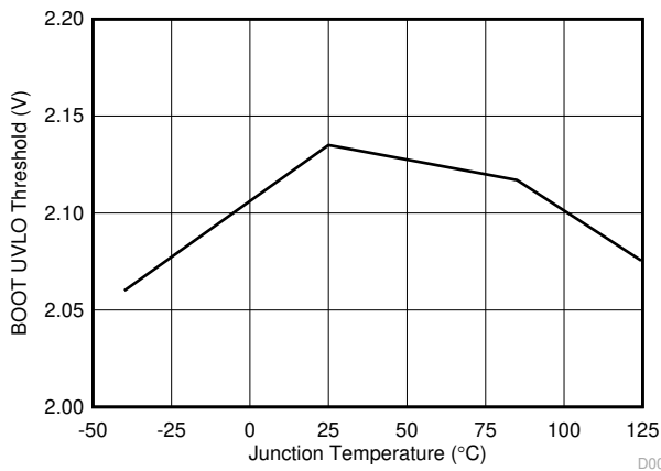
图 5-9. BOOT-SW UVLO 阈值与结温间的关系
