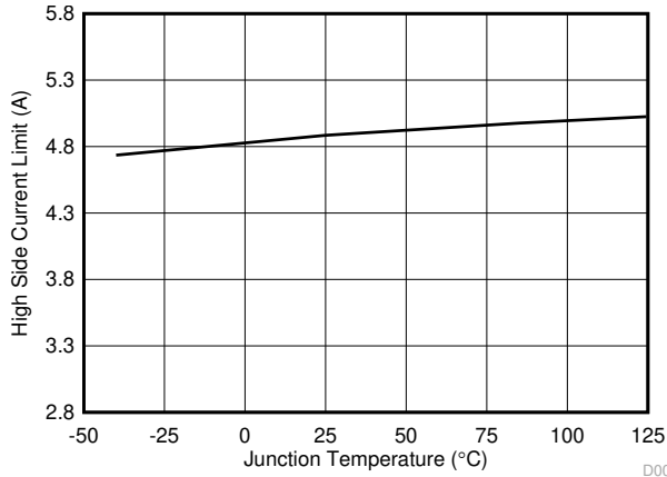
图 5-7. 高侧电流限制阈值与结温间的关系
