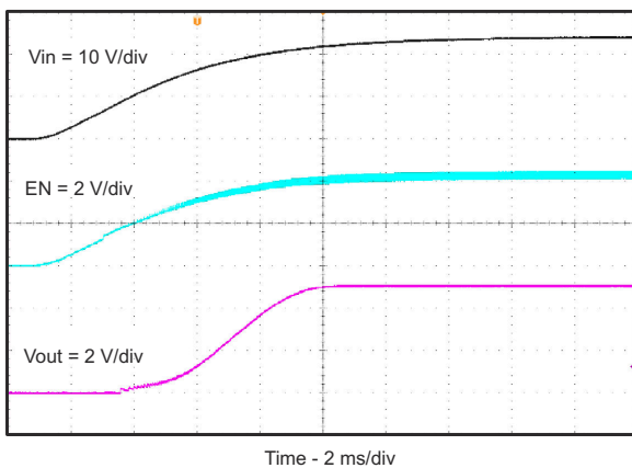
图 7-12. 相对于 VIN 的启动
