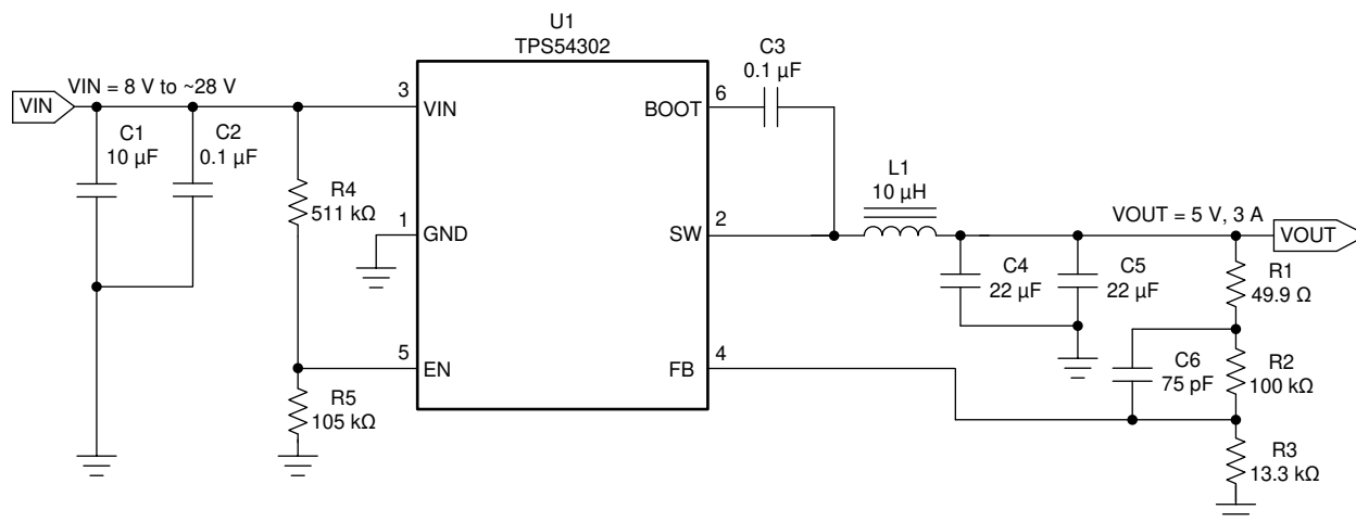
图 7-1. 5V、3A 参考设计
