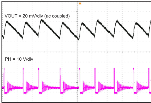
图 7-8. 输出电压纹波
