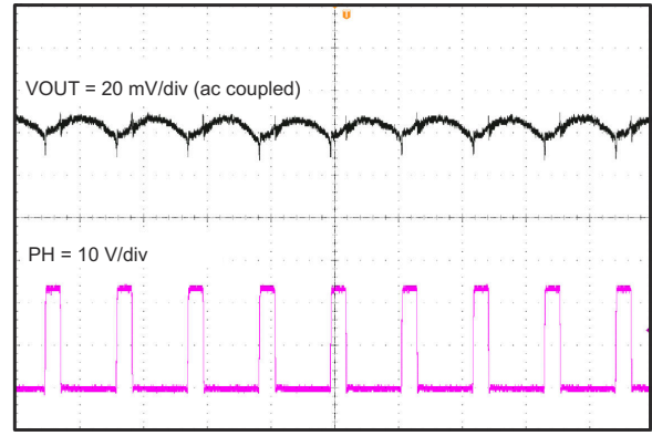
图 7-9. 输出电压纹波
