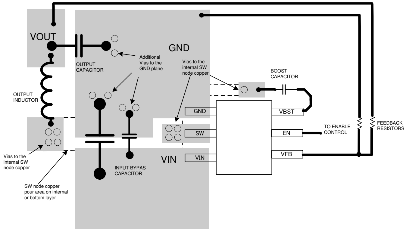
图 7-16. 电路板布局
