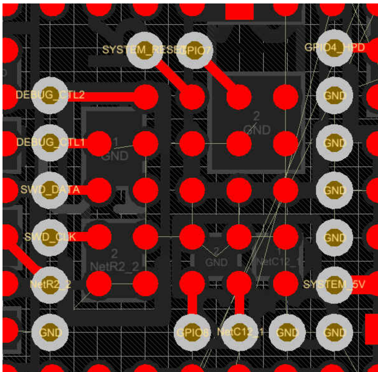
图 12-15. Void Via Placement
