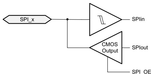
图 9-52. IOBUF_GPIOHSSI
