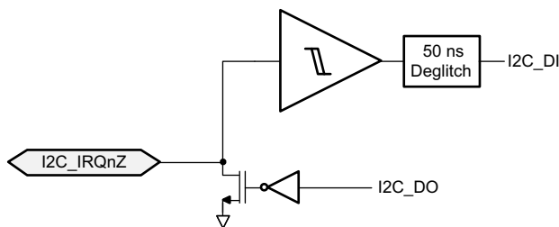
图 9-51. IOBUF_I2C I/O
