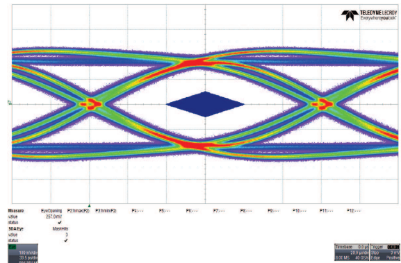
图 14. Downstream Port 1
