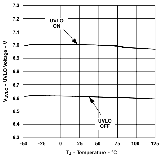
图 7-9. 欠压锁定与温度间的关系
