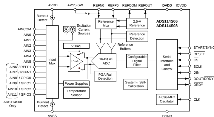
功能方框图
