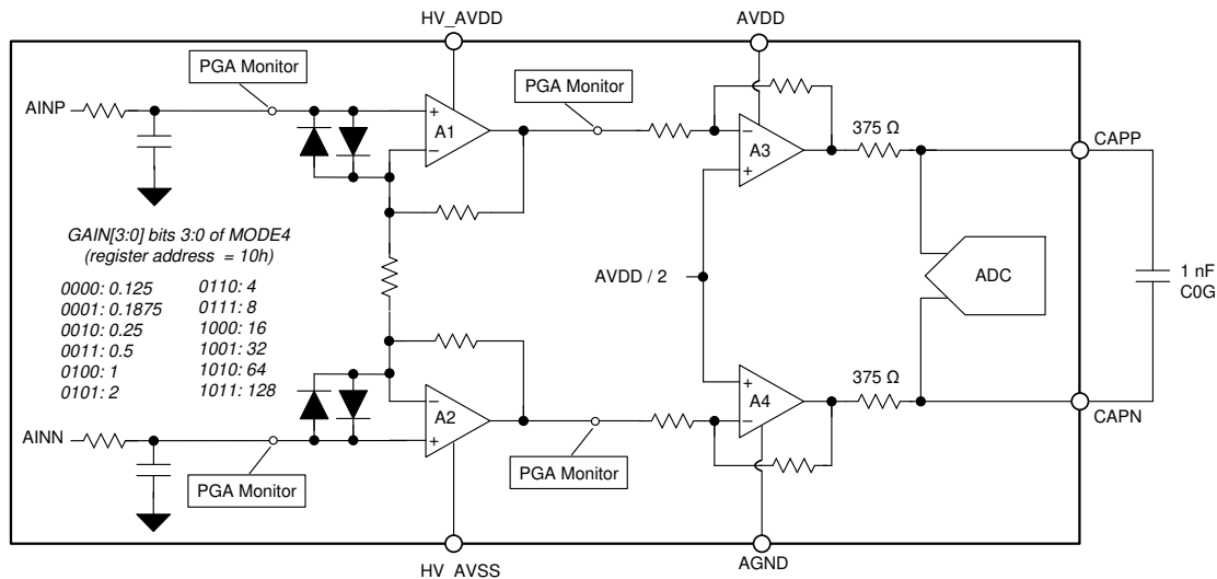
图 9-1. PGA Block Diagram
