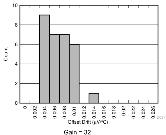
图 7-15. Offset Error Drift Distribution
