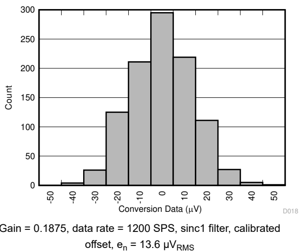
图 7-8. Conversion Data Distribution
