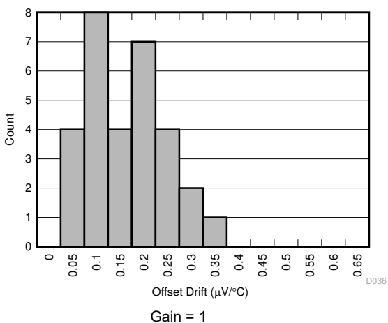
图 7-14. Offset Error Drift Distribution
