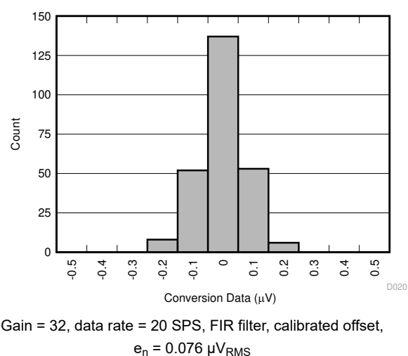
图 7-9. Conversion Data Distribution
