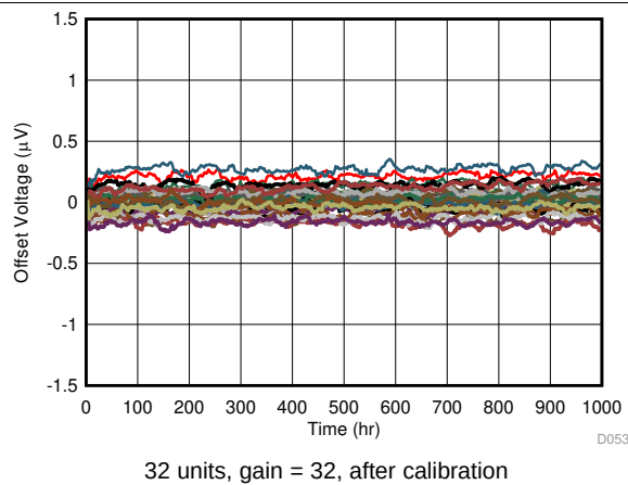
图 28. Offset Voltage Long-Term Drift
