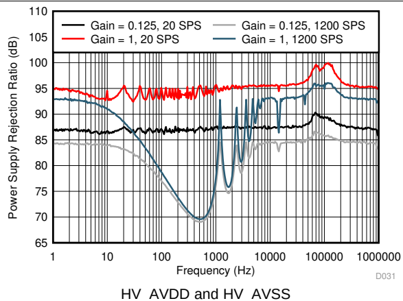
图 49. PSRR vs Frequency
