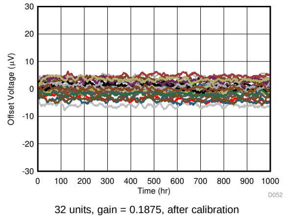
图 27. Offset Voltage Long-Term Drift
