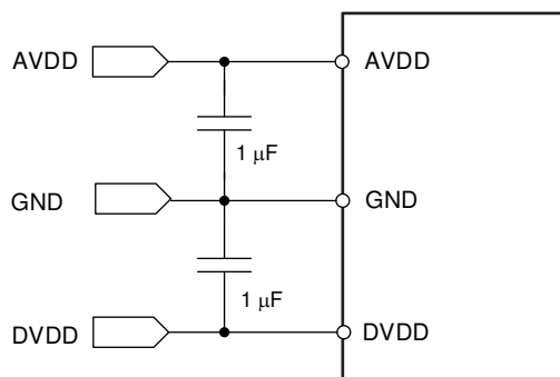
图 8-3. Power-Supply Decoupling
