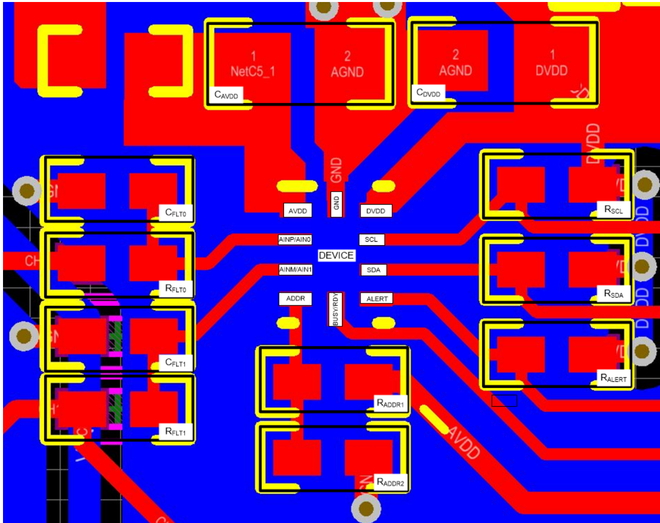
图 124. Example Layout
