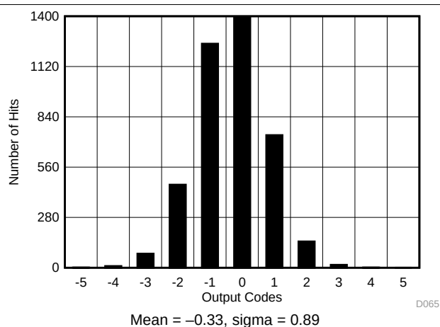
图 75. DC Histogram for OSR16
