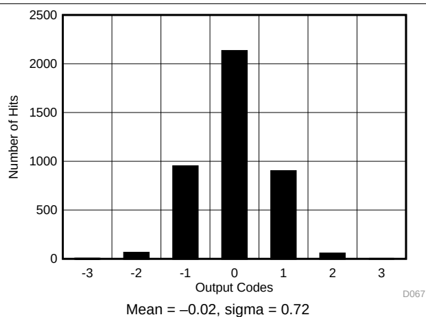
图 77. DC Histogram for OSR64
