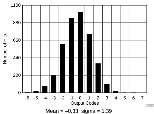
图 73. DC Histogram for OSR4
