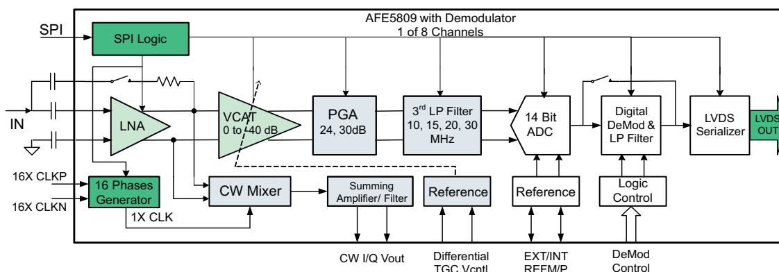
图 1. 方框图
