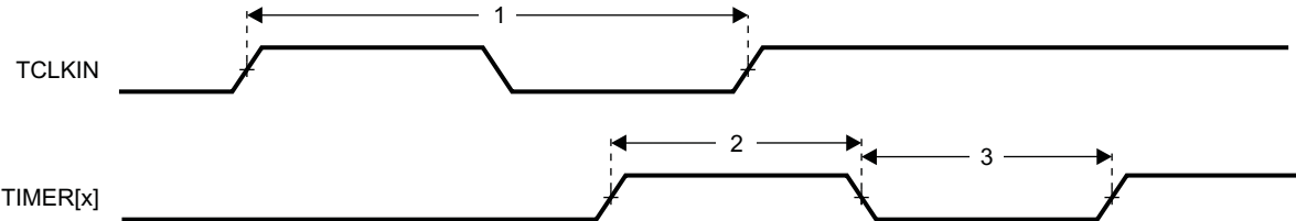
图 7-2. Timer Timing
