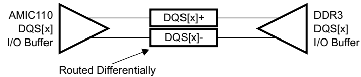
图 7-62. DQS[x] Topology
