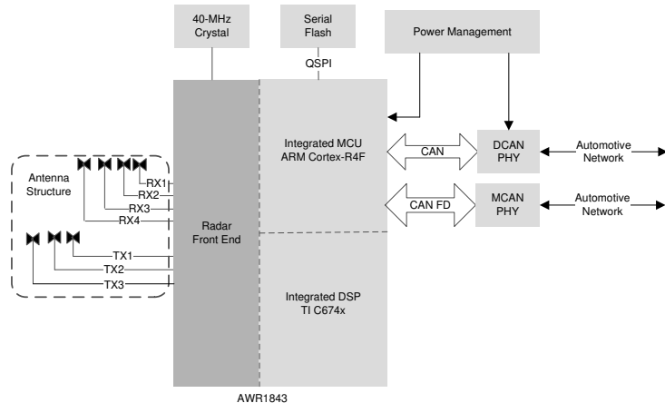
图 2-1. 适用于汽车应用的自主雷达传感器
