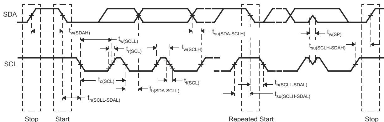
图 7-14. I2C 时序图
