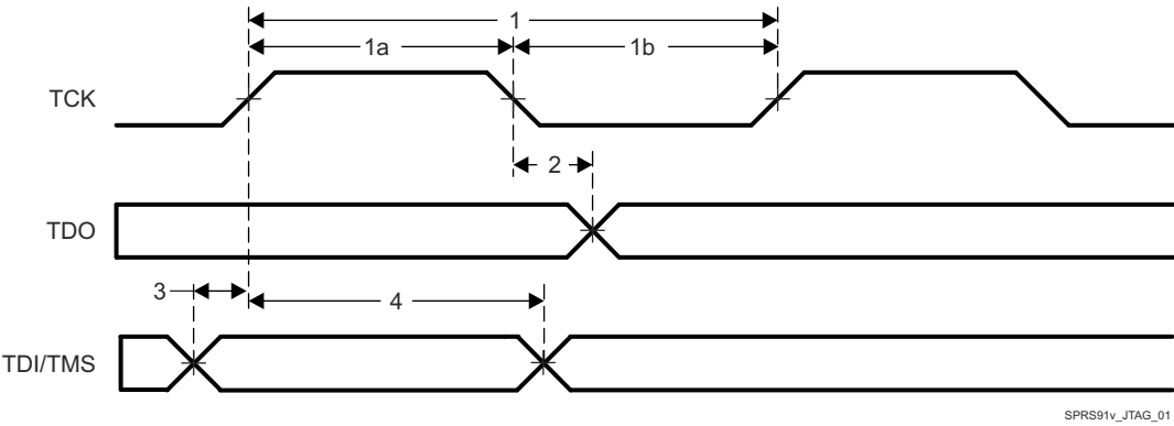
图 7-21. JTAG 时序
